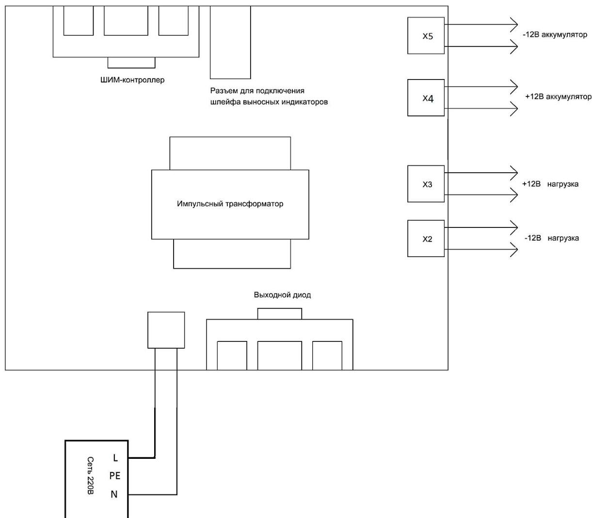
Рис. 1 Схема подключения
